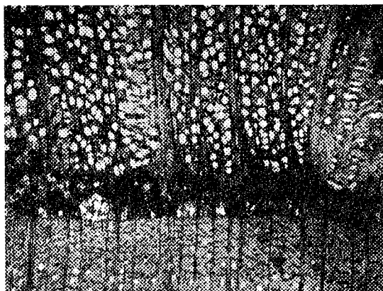
Slika 1: Bukev ( Fagus sylvatica L.), prečni prerez: neposreden odziv kambija na poškodovanje v proksimalnem delu poškodbe ("barierna cona").
