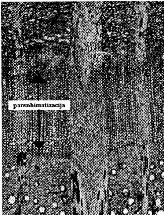
Slika 4: Bukev ( Fagus sylvatica L.), prečni prerez: neposreden odziv kambija na poškodovanje na lokaciji pod poškodbo, ki se kaže v izraziti parenhimatizaciji.
