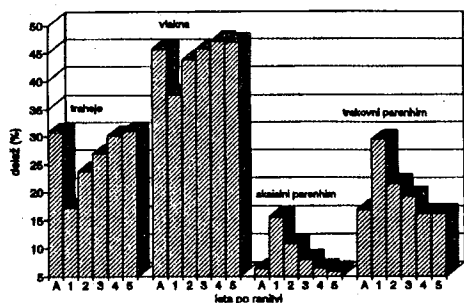
Slika 10: Bukev ( Fagus sylvatica L.): delež posameznih tipov celic v ranem lesu adultnega lesa (A), nastalega tik pred poškodbo (1986) in poranitvenega lesa (1 - 5). Rezultati so povprečja meritev na 12 testnih drevesih.
