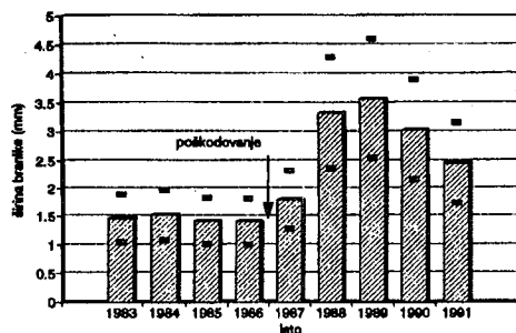
Slika 11: Bukev ( Fagus sylvatica L.): povprečne širine branjke v lesu, nastalem pred in po poškodovanju. Rezultati so povprečja meritev na 12 testnih drevesih.
