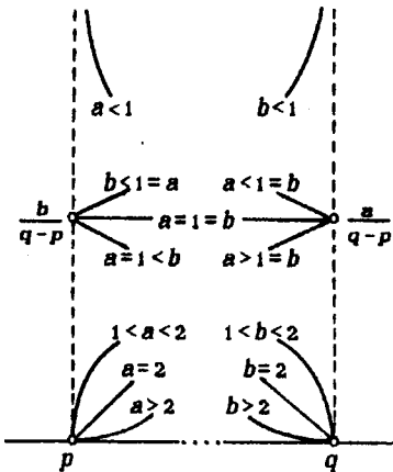
Slika 1 Gostota porazdelitve B_1(p, q, a, b)
