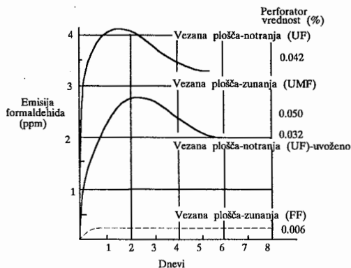
Slika 1: Emisija prostega formaldehida iz različnih tipov vezanih plošč (05/16)
