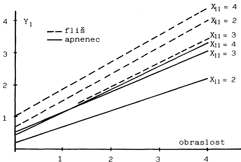
Diagram 1 Stopnja erozije ( y_1 ) v odvisnosti od obraslosti po podlogah in trdotah vlak
