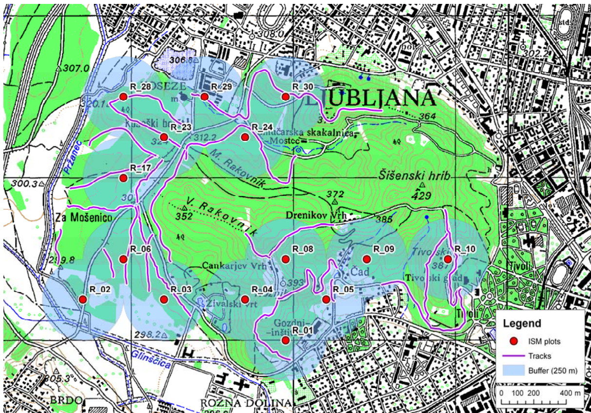
Slika 33. ISM popisne ploskve (ISM plots) in UFMO poti (UFMO tracks) na Rožniku v Ljubljani, kjer smo popisovali škodljive dejavnike. (Pripravil: Nikica Ogris)
