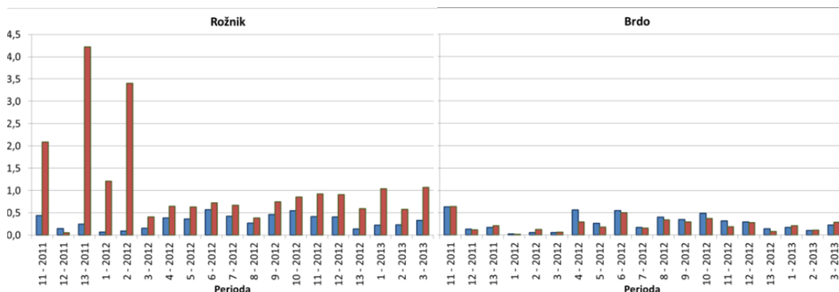
Slika 40. Depozit žvepla v sulfatni obliki na prostem (modri stolpci) in v sestoju (rdeči stolpci) na ploskvah Rožnik in Brdo (v kg S/ha). (Izdela: Daniel Žlindra)
