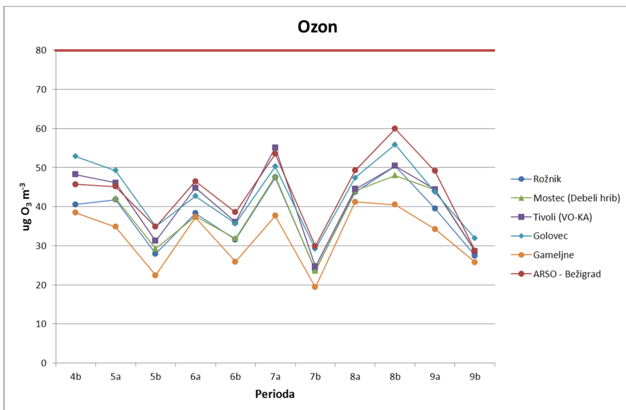
Slika 34. Koncentracije ozona na EMonFUr ploskvah Rožnik v letu 2013. Rdeča črta predstavlja mejo AOT 40. (Izdelal: Daniel Žlindra)
