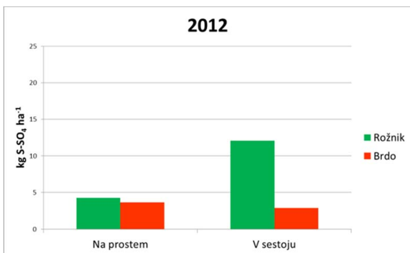
Slika 43. Razmerje depozita žvepla v obliki sulfata na prostem in v sestoju na ploskvah Rožnik in Brdo. (Izdelal: Daniel Žlindra)
