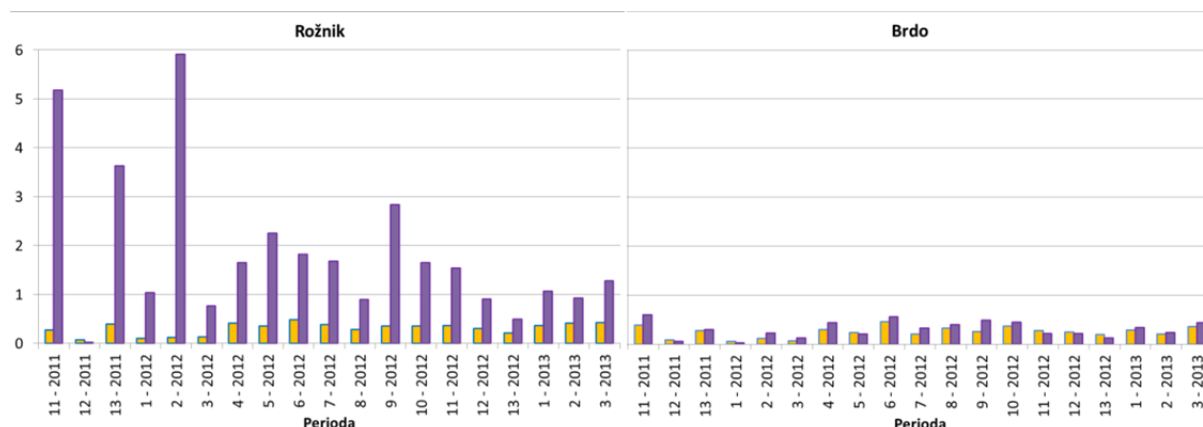
Slika 39. Depozit dušika v nitratni obliki na prostem (rumeni stolpci) in v sestoju (vijolični stolpci) na ploskvah Rožnik in Brdo (v kg N/ha). (Izdelal: Daniel Žlindra)
