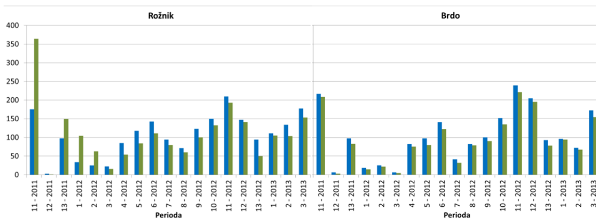
Slika 37. Količina padavin na prostem (modri stolpci) in v sestoju (zeleni stolpci) na ploskvah Rožnik in Brdo (v L/m 2 ). (Izdelal: Daniel Žlindra)
