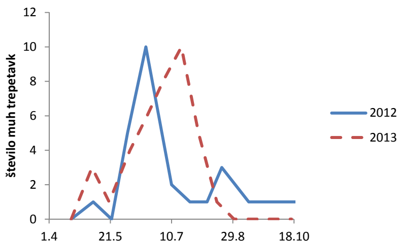
Slika 31: Število muh trepetavk ujetih v malaisove pasti na območju Rožnika v letih 2012 in 2013. Na osi x je prikazan datum v letu. (Izdelal: Maarten de Groot)
