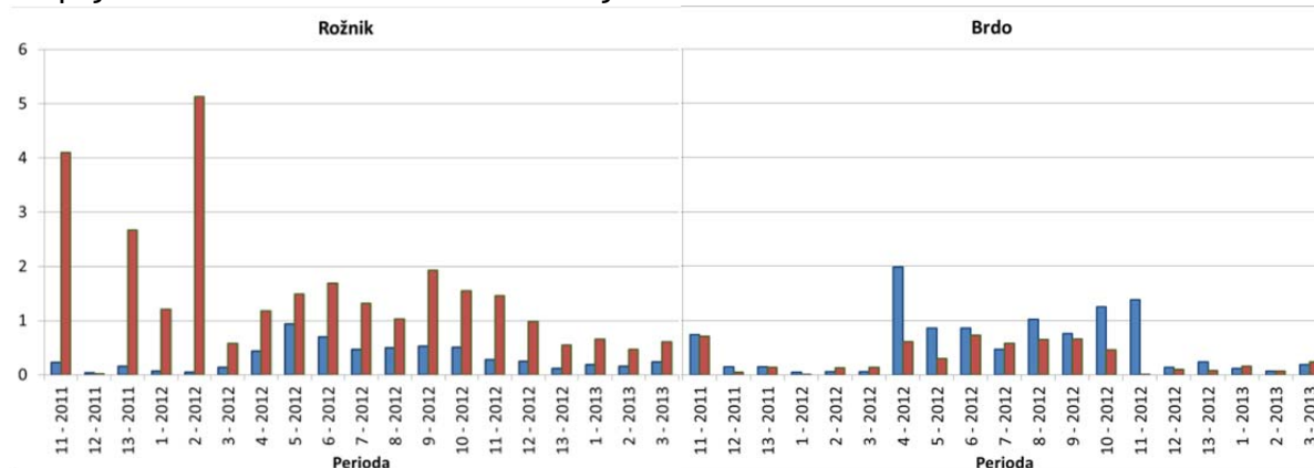
Slika 38. Depozit dušika v amonijevi obliki na prostem (modri stolpci) in v sestoju (rdeči stolpci) na ploskvah Rožnik in Brdo (v kg N/ha). (Izdelal: Daniel Žlindra)
