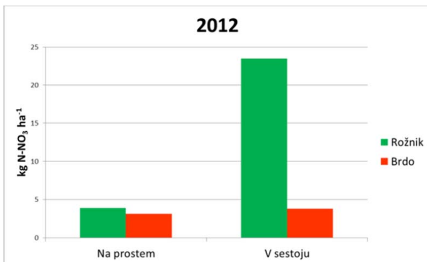
Slika 42. Razmerje depozita dušika v obliki nitrata na prostem in v sestoju na ploskvah Rožnik in Brdo. (Izdelal: Daniel Žlindra)
