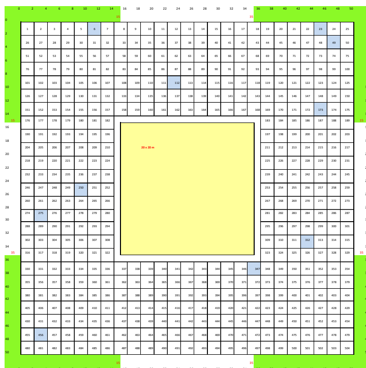
Slika 9. Razporeditev srednje in malih vegetacijskih ploskev na monitorinški ploskvi Rožnik v Ljubljani. (Pripravi: Matej Rupel)
