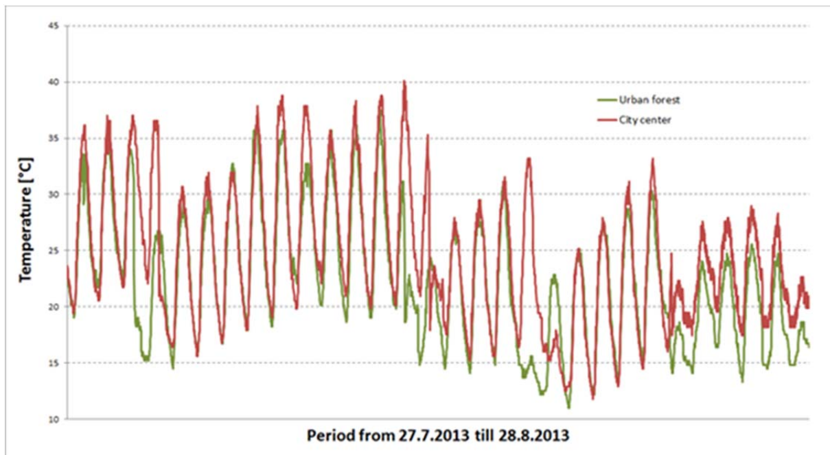
Slika 6. Poletne temperature zraka v centru Ljubljane. (Izdelal: Mitja Ferlan)
