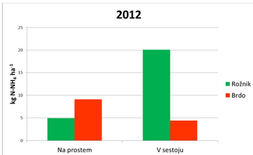
Slika 41. Razmerje depozita dušika v obliki amonija na prostem in v sestoju na ploskvah Rožnik in Brdo. (Izdelal: Daniel Žlindra)
