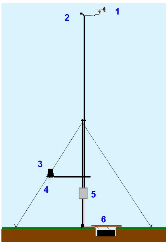
Slika 5. Shema samodejnih meteoroloških postaj postavljenih v okviru projekt (1 – Merilnik hitrosti vetra, ki beleži tudi smer vetra (Davis Instruments), 2 – Merilnik Sončevega sevanja (Davis Instruments), 3 – Merilnik padavin (Davis Instruments), 4 – Samodejni registrator temperature in relativne zračne vlage (Votcraft DL-120TH), 5 – Omarica z merilnikom zračnega pritiska (Freescale Semiconductor) in s hranilnikom podatkov, ki shranjuje podatke o padavinah, Sončevem sevanju, zračnem tlaku in vetru (Campbell Scientific datalogger CR200), 6 – Glavna baterija). (Pripravil Mitja Ferlan)
