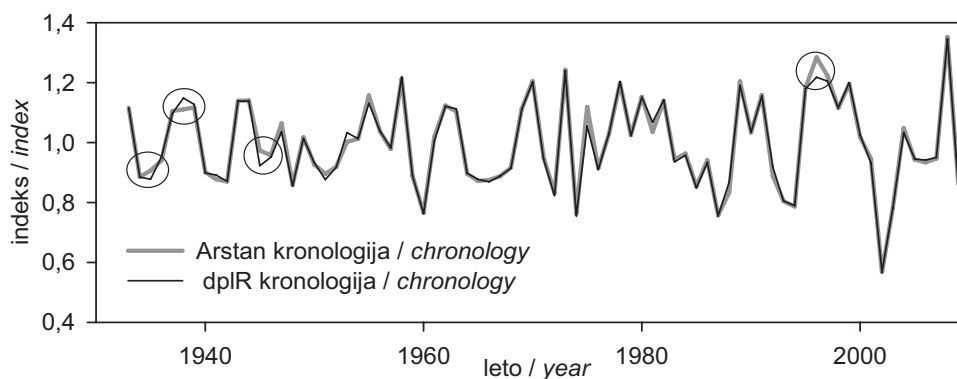
Slika 6: Primerjava kronologij STD, izdelanih v ARSTAN-u in dplR
