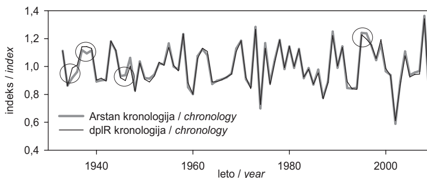
Slika 7: Primerjava kronologij RES, izračunanih v ARSTAN-u in dplR
