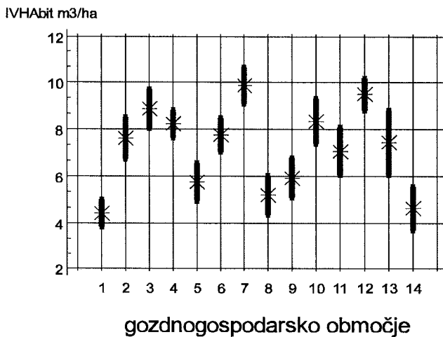
Slika 10: Ocena prirastka lesne zaloge po gozdnogospodarskih območjih z mejami zaupanja.
