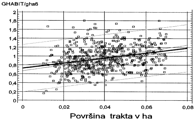
Slika 2: Povezava med površino trakta in razmerjem ocen temeljnice s kotnoštevno metodo in modificirano metodo 6-dreves.
