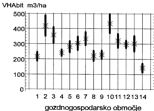
Slika 9: Ocena lesne zaloge po gozdnogospodarskih območjih z mejami zaupanja.
