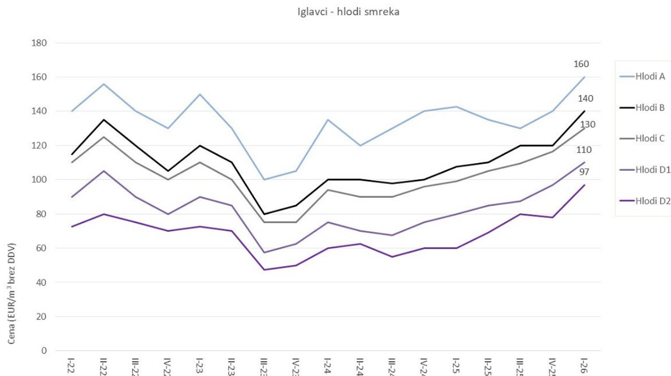
Slika 2: Odkupne cene hlodov smreke iz zasebnih gozdov od leta 2022 dalje (cene so podane v EUR/m 3 brez DDV na kamionski cesti)
