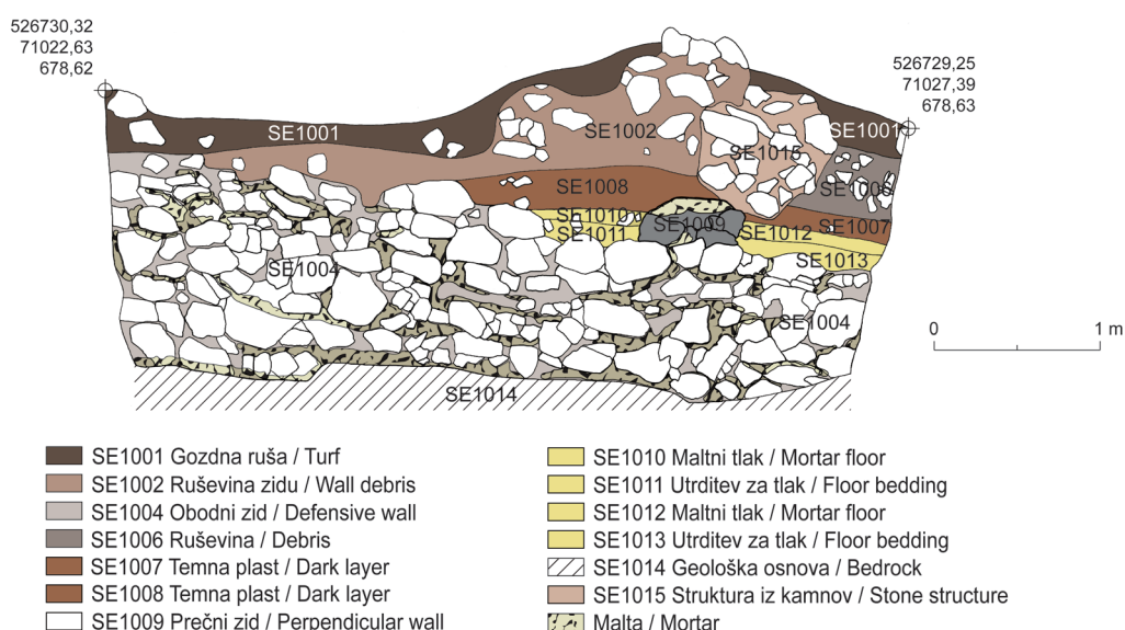
Sl. 8: Zidani gaber. Sonda 1, risba zahodnega profila. Vzhodni obodni zid, na katerega se naslanja prečni zid. Ob tem sta dva apnena tlaka, ki ju prekrivajo temna plast in plasti ruševine. (koordinatni sistem D96/TM)
