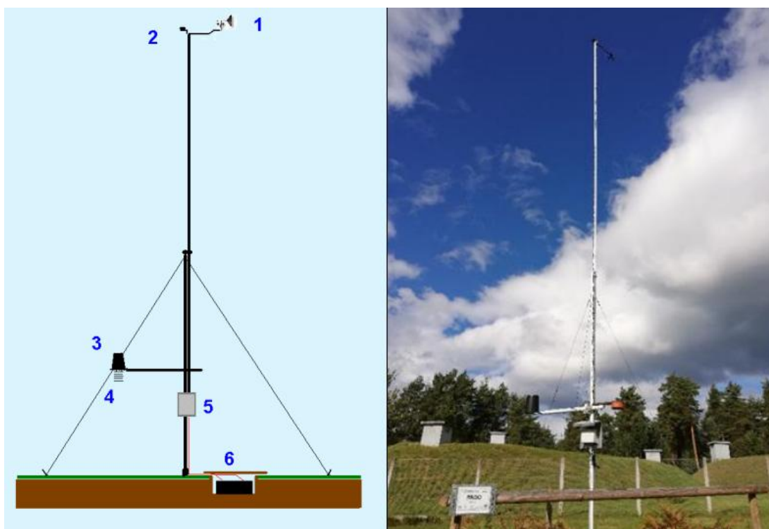
Slika 68: Skica in slika samodejne meteorološke postaje Gozdarskega inštituta Slovenije na Brdu pri Kranju (Skica: I. Sinjur, Foto: M. Rupel)
