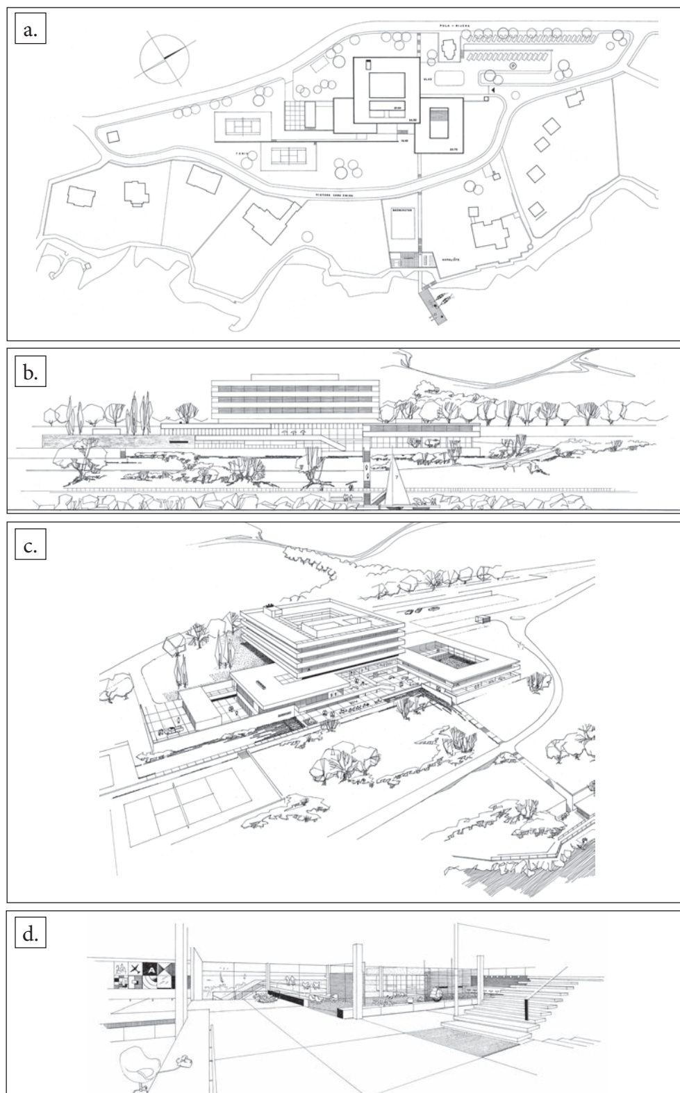
Slika 4: Lovran, hotel, natječajni projekt (1960.): a) situacija, b) pročelje prema moru, c) perspektiva sklopa, d) perspektiva interijera (HAZU-HMA Dragomanović, AD/9/9; HAZU-HMA Nikšić, RN/3/28).
