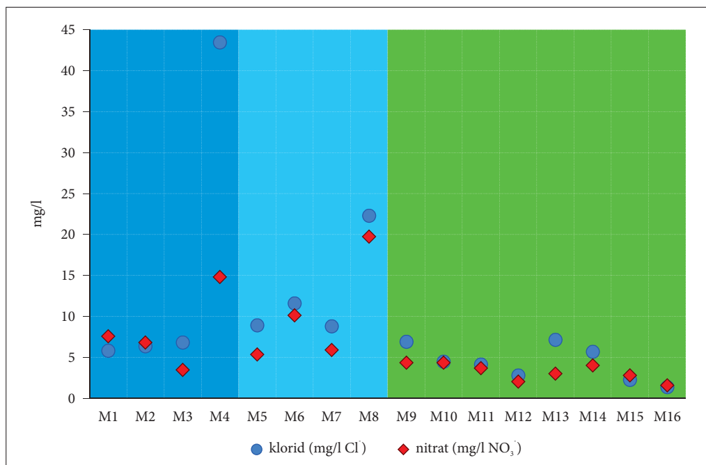
Slika 5: Povprečne vrednosti klorida in nitrata na vzorčnih mestih.
