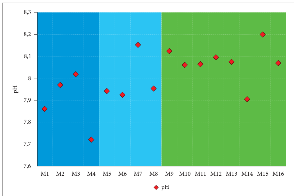
Slika 4: Povprečne vrednosti pH na vzorčnih mestih.
