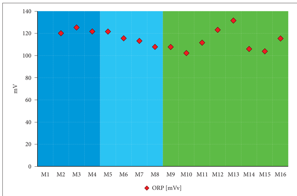
Slika 8: Povprečna vrednost ORP na vzorčnih mestih.
