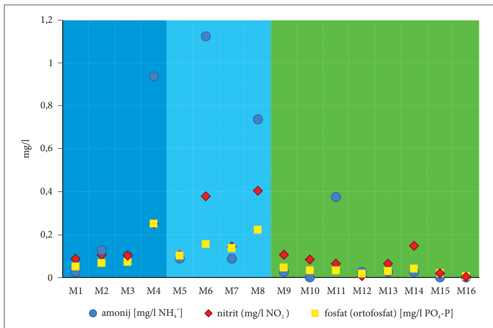
Slika 6: Povprečne vrednosti nitrita, amonija in fosfata na vzorčnih mestih.
