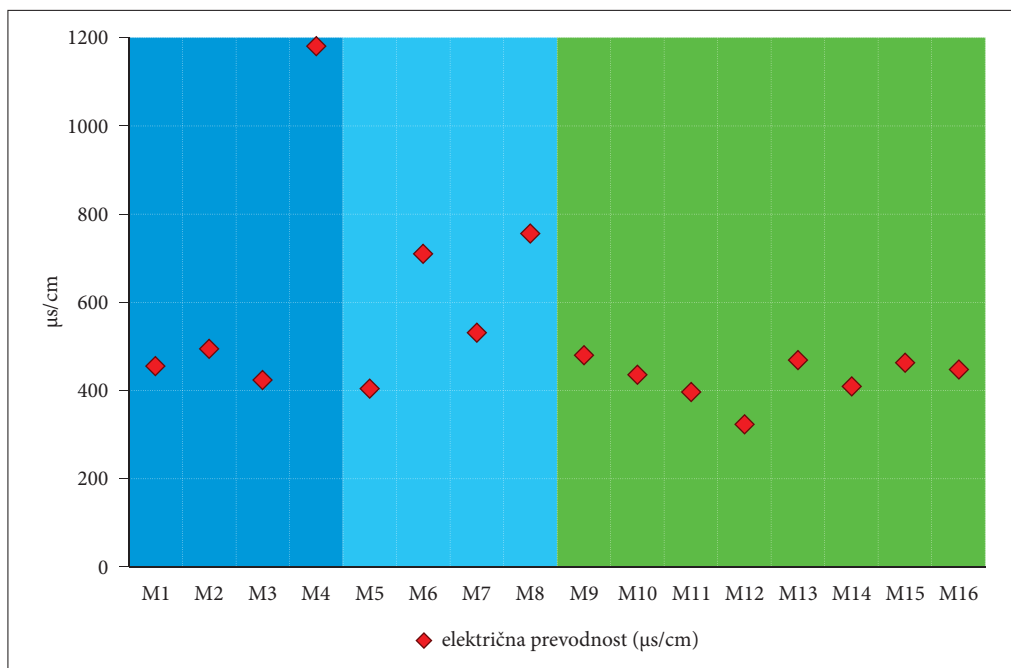
Slika 10: Povprečna vrednost SEP na vzorčnih mestih.
