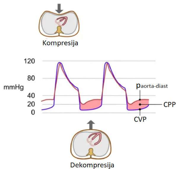
Slika 1. Perfuzijski tlak skozi koronarne arterije (CPP) med kardio-pulmonalnim oživljanjem. CVP, centralni venski tlak; p aorta-diast , tlak v aorti med dekompresijo (analogen tlaku v diastoli).
