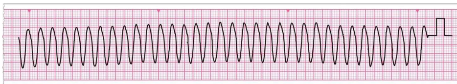
Slika 4. Zapis ventrikularne tahikardije na elektrocardiogramu.
