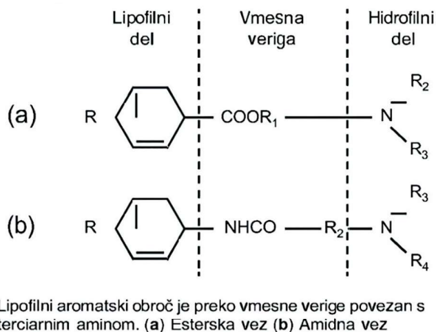
Slika 1. Splošna struktura estrskih in amidnih lokalnih anestetikov. Povzeto po: Perrin in sod. Anaesth Intens Care Med , 2022.
