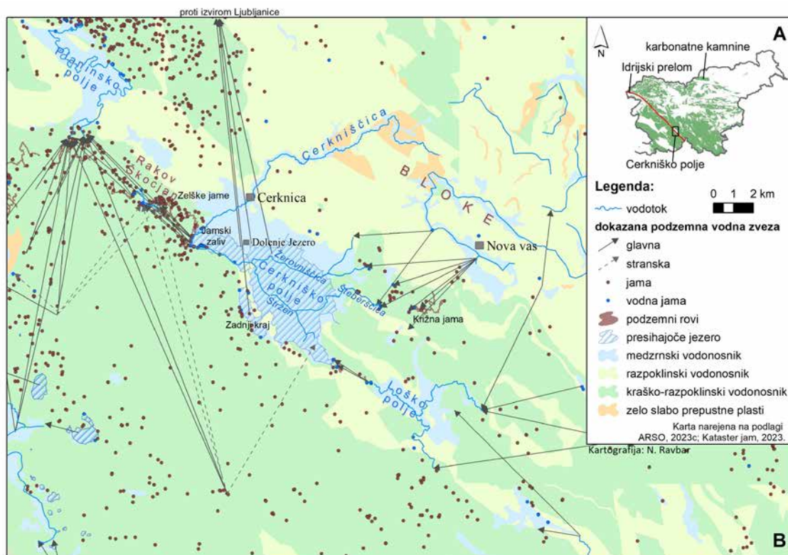
Slika 2: Potek Idrijske prelomne cone (A) ter hidrogeološke in speleološke razmere Cerkniskega polja in okolice (B).
