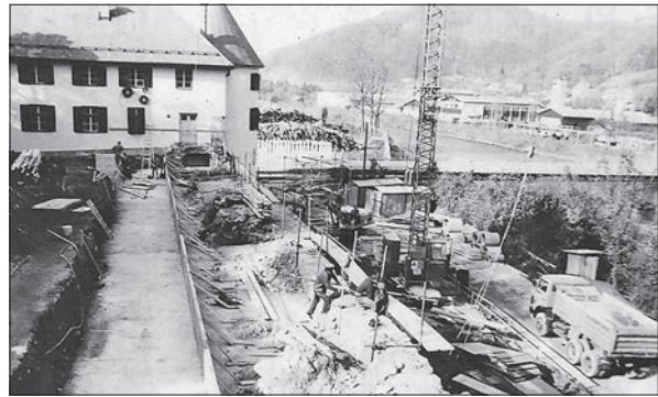
Pogled na začetek gradnje nadomestnega severnega trakta leta 1990 (fotografija iz zasebne dokumentacije Igorja Sapača).
