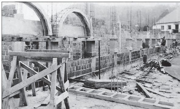
Gradnja pritličnih arkad nadomestnega severnega trakta leta 1990 (fotografiji iz zasebne dokumentacije Igorja Sapača).
