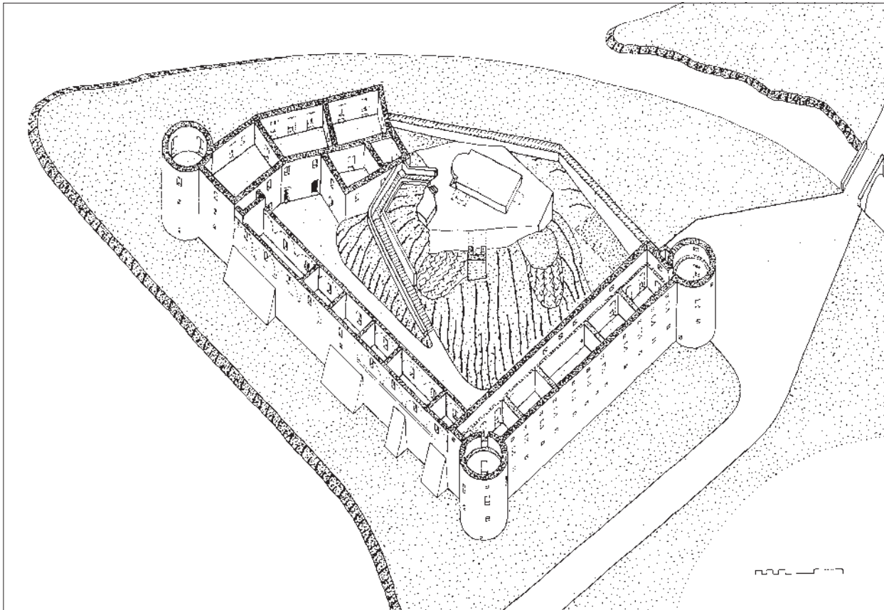
Grad Vrbovec okoli leta 1945. Poskus rekonstrukcije. Aksonometrična študija (risal: Igor Sapač, 2023 in 2025).
