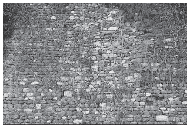
Detajl zidovja na jugovzhodni strani nekdanjega grajskega jedra (foto: Igor Sapač, 2016).
