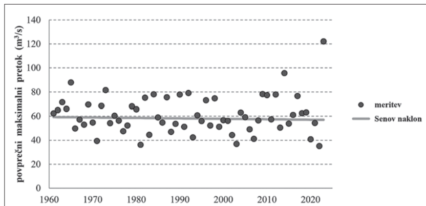
Slika 7: Trend povprečnih maksimalnih letnih pretokov Savinje na vodomerni postaji Nazarje v obdobju od 1961 do 2023.
