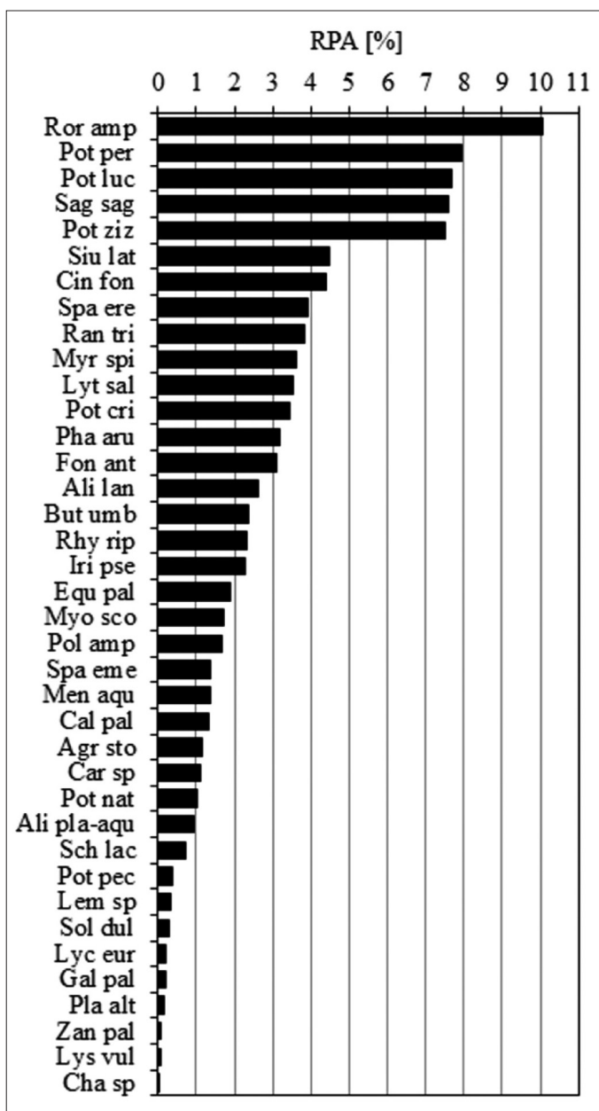
Slika 7: Relativna rastlinska abundanca (RPA) posameznega taksona - razmerje abundance posameznega taksona (ocenjena z lestvico od 1 do 5), glede na celokupno pojavljanje vseh taksonov v reki.
