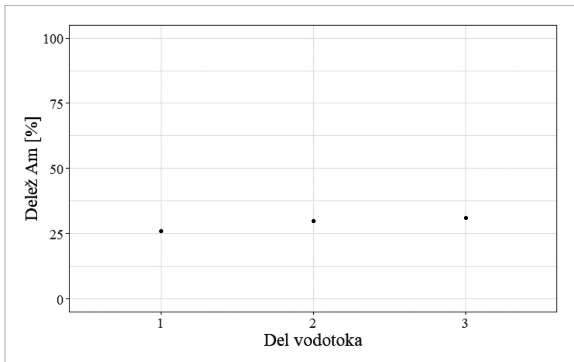
Slika 4: Delež amfibijskih vrst (Am), prisotnih v prvem (od 1. do 5. rečnega oseka), drugem (od 6. do 10. odseka) in tretjem (od 11. do 15. odseka) delu reke Rak. Vz dolž reke se je delež amfibijskih vrst s 26,0 % povečal na 30,0 % in 31,0 %.
