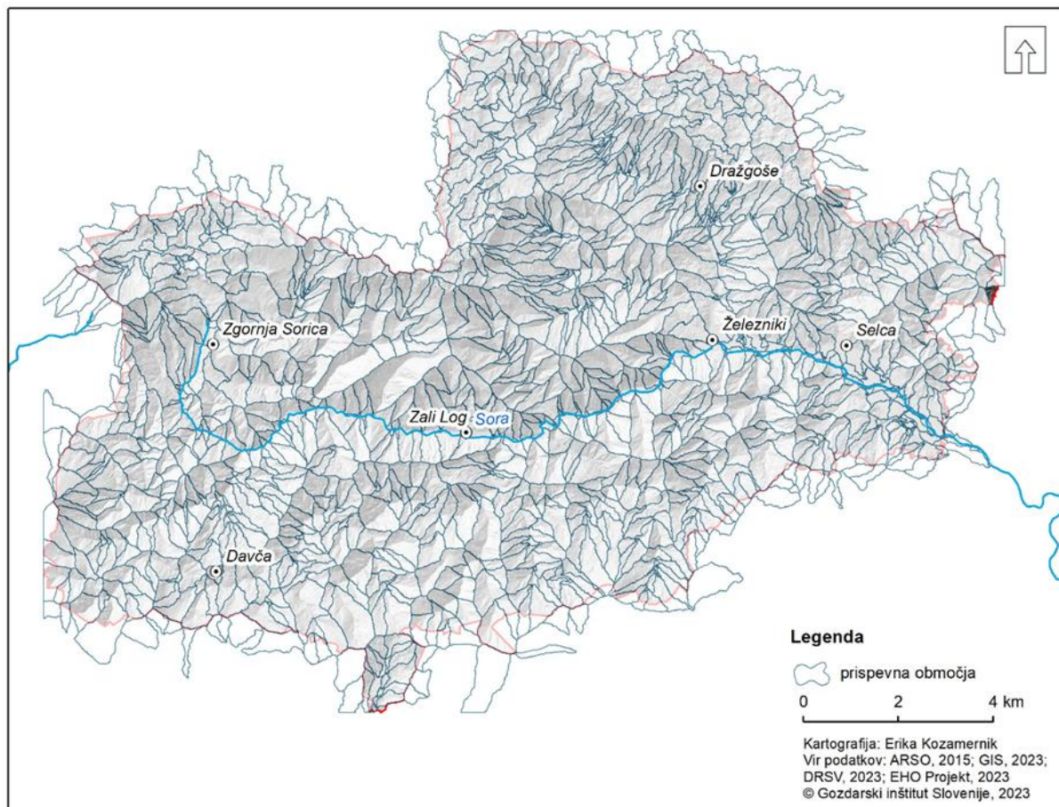
Slika 9: Prispevna območja hudournikov, generirana s programom ArcGIS Pro 3.1.0. z orodji Arc Hydro (ESRI, 2022) na primeru občine Železniki.
