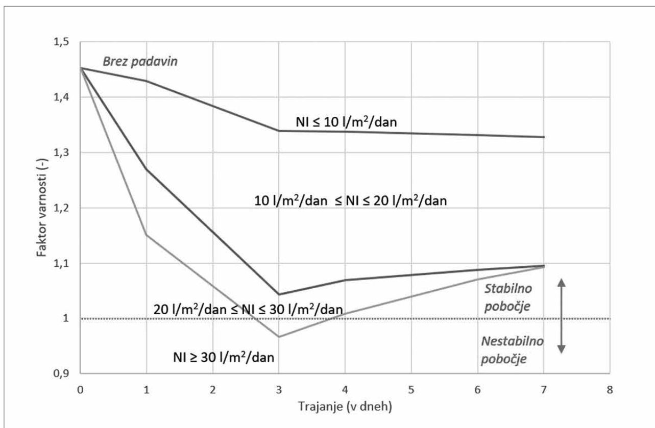
Slika 6: Vpliv infiltracije vode v pobočje na časovni razvoj faktorja varnosti na stabilnost, pri hkratnem nižanju strižne trdnosti zemljine (ilustracija: avtorji)
