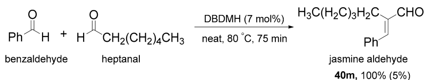
Scheme 2. Synthesis of (E)-2-benzylideneheptanal (jasmine aldehyde).
