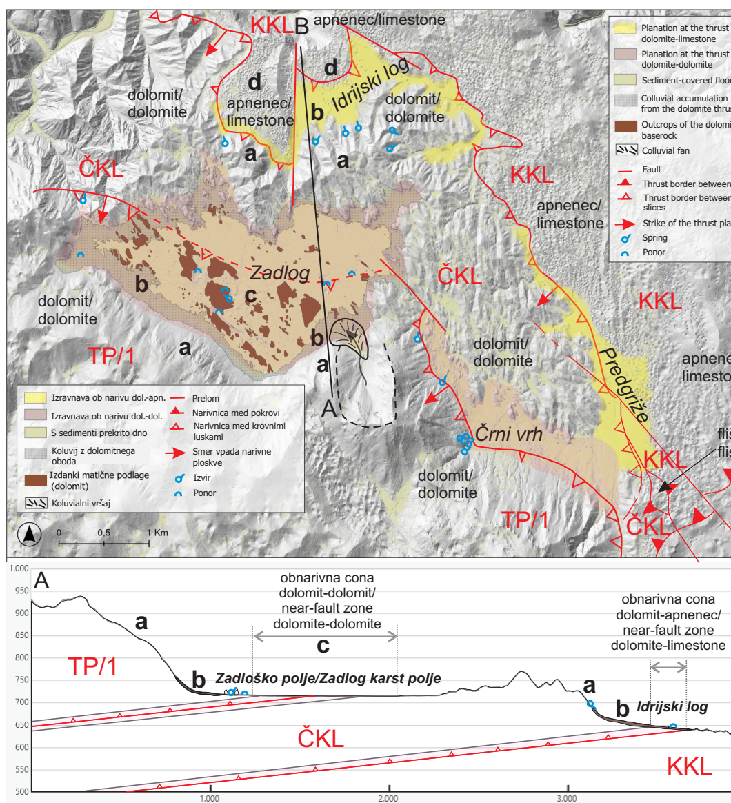
Fig. 8. Thrust-shear surface morphology. Sl. 8. Obnarivna morfologija površja.
