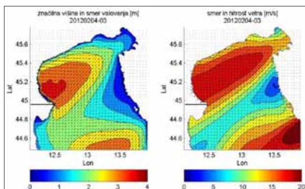
Slika 3: Rezultati valovnega modela SWAN, ki omogoča napoved značilne smeri in višine valovanja v Tržaškem zalivu. Na sliki so prikazane značilna višina in smer valovanja (levo) ter smer in hitrost vetra (desno). Na abscisni osi so navedene geografske dolžine, na ordinatni pa geografske širine v stopinjah.
