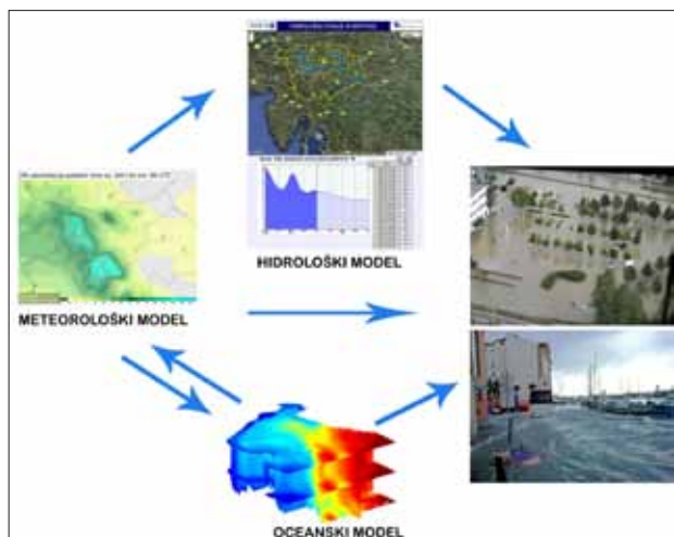
Slika 1: Komunikacija med numeričnimi modeli v dvosmerno sklopljeni modelski verigi. Oceanski in atmosferski model si vzajemno pošiljata robne pogoje med integracijo. Kakovostna napoved stanja morja vodi do kakovostnejše napovedi vremena in tako do boljše hidrološke napovedi.
