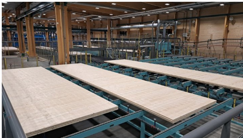
Slika 7: Tehnološka linija v podjetju Stilles, za proizvodnjo križno lepljenih plošč
