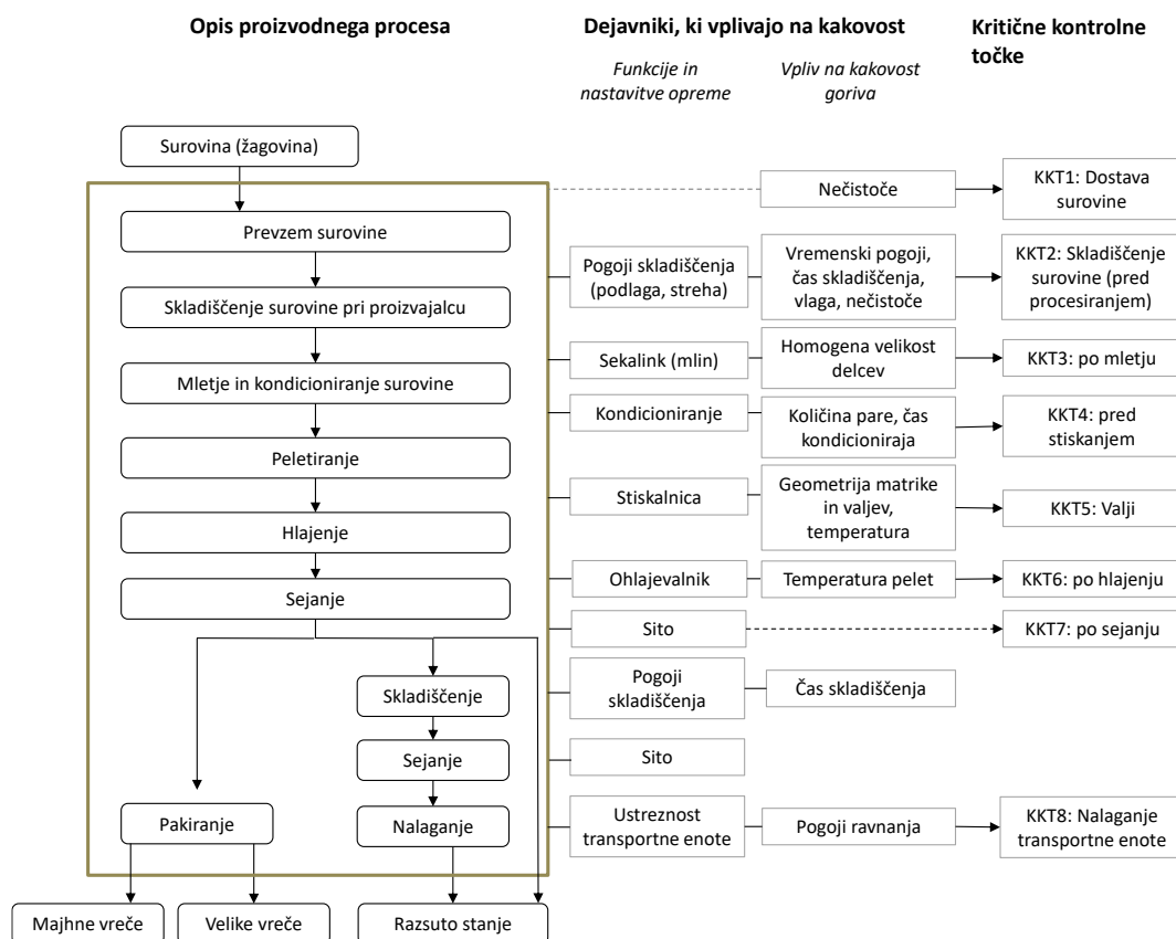
Slika 3: Primer shematskega prikaza proizvodnega procesa s kritičnimi kontrolnimi točkami (KKT).
