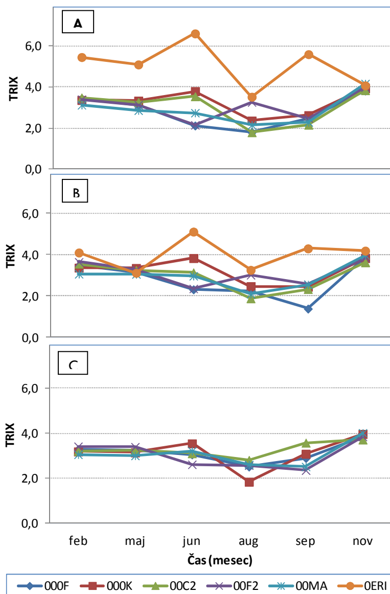
Slika 8. Prikaz vrednosti TRIX indeksa evτροφikacijskega monitoringa v obalnem morja R Slovenije (A - globina 0,3 m; B- globina 5m; C - globina 10 ali 15 m).
