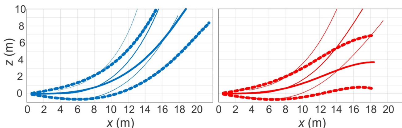
SLIKA 7. ZAČETNO REDČENJE PRI IZPUSTU. DEBELE ČRTE PRIKAZUJEJO RAZŠIRJANJE VZGONSKEGA CURKA IZ DIFUZORSKE ODPRTINE, TANKE ČRTE PA IZ IZPUSTNE CEVI BREZ DIFUZORJA. MODRE ČRTE PRIKAZUJEJO RAZŠIRJANJE CURKA V ZIMSKEM ČASU, RDEČE PA V POLETNEM ČASU. ČRTKANE ČRTE PRIKAZUJEJO 'OVOJNICO' VZGONSKEGA CURKA, NA KATERI JE HITROST CURKA 1/E (=0,37) HITROSTI V SREDICI.
