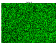
(b-Na)
