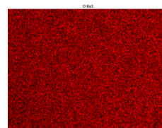
(b-O)
