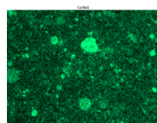
(b-Ca)
