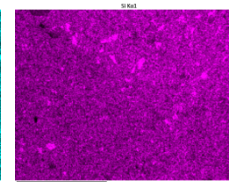
(b-Si)
