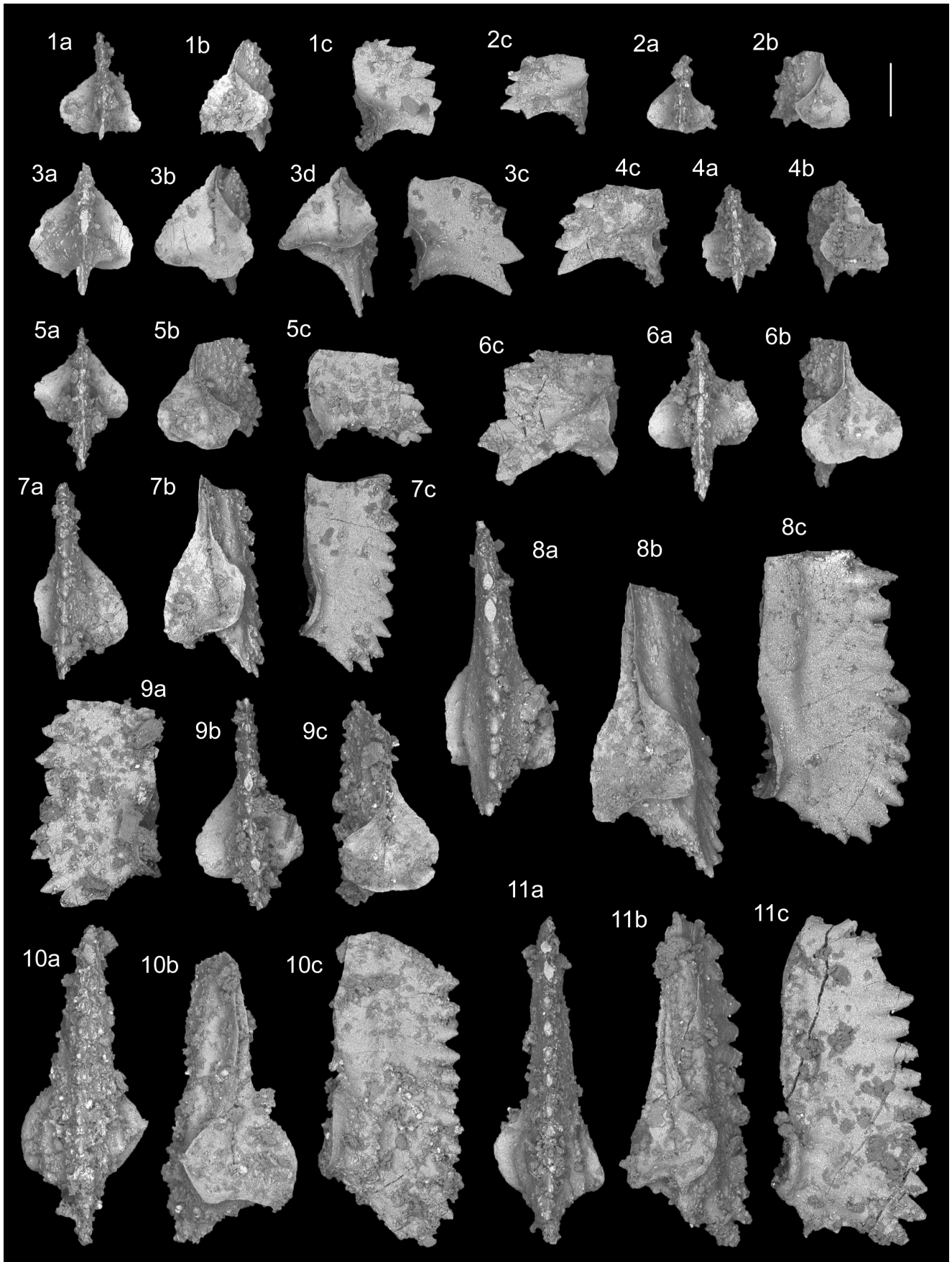
Fig. 8 - SEM images of conodonts from the Tulcea Veche locality, sample TV 110a (GeoZS 6168). 1–3, 5) Triassospathodus sp.; 4) Triassospathodus hungaricus (Kozur & Mostler); 6) Triassospathodus ex gr. hungaricus (Kozur & Mostler); 7, 9) Triassospathodus symmetricus (Orchard); 8, 10–11) Icriospathodus crassatus (Orchard). Scale bar: 100 microns; a) upper, b) lower, c) lateral view.
