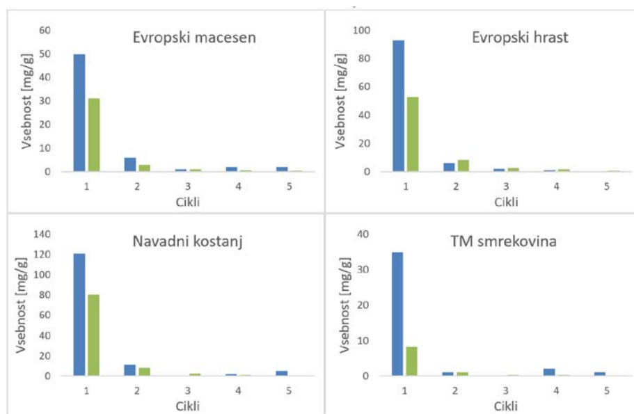
Slika 1: Vsebnost celokupnih ekstraktivov na gram absolutno suhega lesa (mg/g dw) (modri stolpci) in vsebnost celokupnih fenolov v ekvivalentih galne kisline na gram absolutno suhega lesa (mg GAE/g dw) (zeleni stolpci) v jedrovini evropskega macesna (Ld), evropskega hrasta (Q), navadnega kostanja (Cs) in termično modificirane smrekovine (TERM), pridobljenih v vsakem od petih zaporednih ciklov ekstrakcije z 90-% vodno raztopino metanola na sistemu ASE
