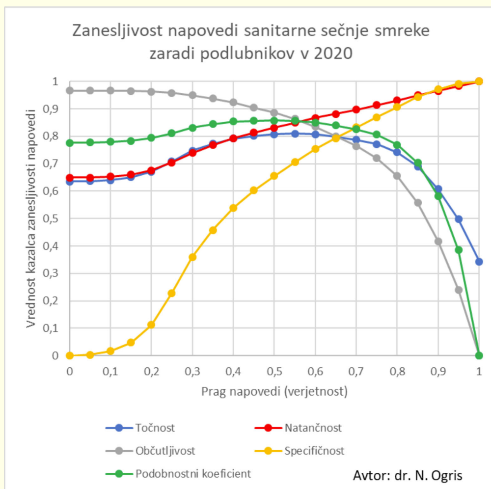
Slika 1: Točnost, natančnost, občutljivost, specifičnost in koeficient podobnosti napovedi sanitarne sečnje smreke zaradi podlubnikov v 2020 glede na različen prag napovedi
