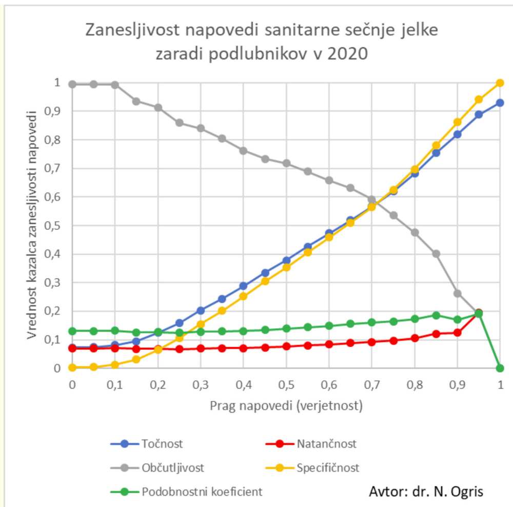
Slika 3: Točnost, natančnost, občutljivost, specifičnost in koeficient podobnosti napovedi sanitarne sečnje jelke zaradi podlubnikov v 2020 glede na različen prag napovedi
