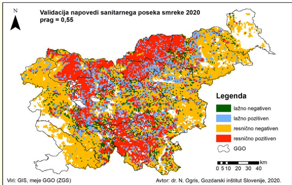
Slika 2: Preverjanje napovedi sanitarne sečnje smreke zaradi podlubnikov v 2020 z upoštevanjem praga 0,55 (verjetnost napovedi)
