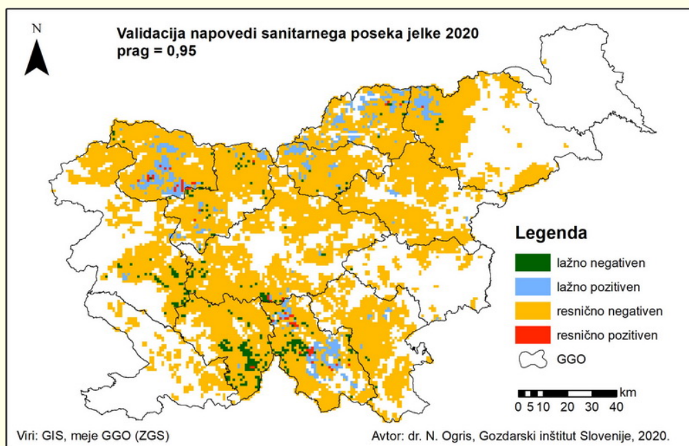
Slika 4: Preverjanje napovedi sanitarne sečnje jelke zaradi podlubnikov v 2020 z upoštevanjem praga 0,95 (verjetnost napovedi)
