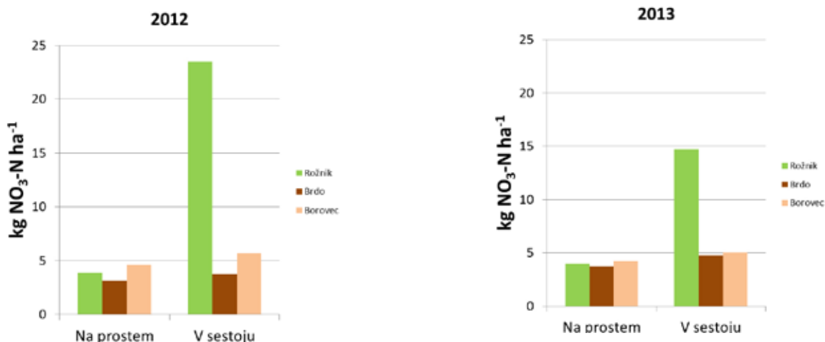
a) b) Slika 6. Primerjava letnih vnosov nitratnega dušika med urbanim gozdom (Rožnik) in ploskvami intenzivnega spremljanja stanja gozdnih ekosistemov zunaj urbanih središč (Brdo, Borovec) v letih a) 2012 in b) 2013 // Figure 6: Comparison of annual deposition of nitrate nitrogen at urban forest monitoring plot Rožnik in Ljubljana and forest monitoring plots Brdo and Borovec in a) 2012 and b) 2013
