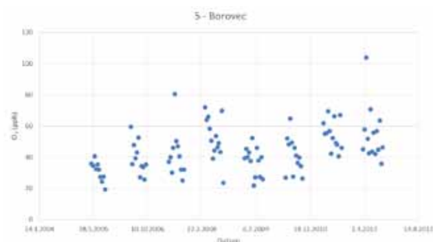
Slika 4. Povprečne 14-dnevne vsebnosti ozona ( \text{O}_3 ) v zraku (ppb) na a) ploskvi intenzivnega spremljanja stanja gozdnih ekosistemov Borovec in b) ploskvi Rožnik v urbanem gozdu v Ljubljani
