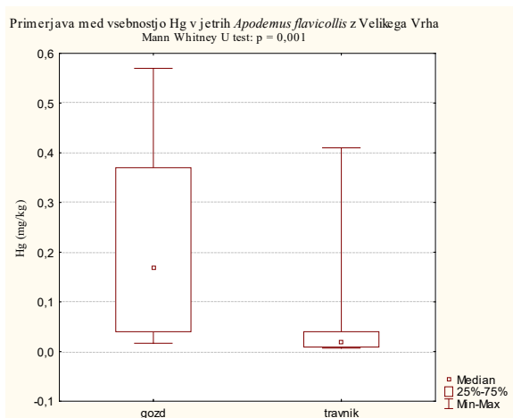
Slika 2: Primerjave vsebnosti Hg in Cd v gozdnih in travniških tleh ter v jetrih rumenogrla miši Apodemus flavicollis , ujetih na območju gozdne in travniške ploskve. Z rdečo linijo smo označili mejno imisijsko vrednost za Hg in Cd (Ur. l. RS, št. 68/1996); z modro črto pa kritično koncentracijo Cd za jetra malih sesalcev (Ma in sod., 1991, Wijnhoven in sod., 2008).
